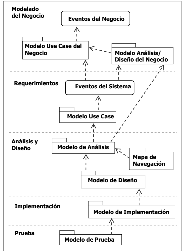
Figura 3: Modelos en RUP-GDIS y sus Dependencias
